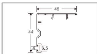
Door Sash Interlock Code: D058 Weight (kg/m): 0.19 Pcs/Bag : 20
